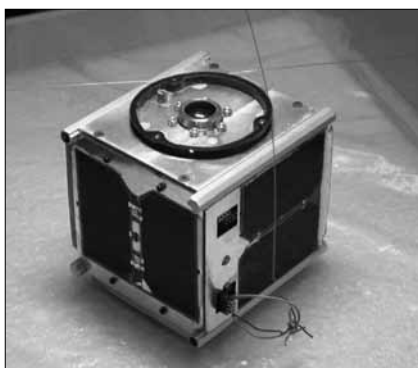
AAU cubesat (Ун-тет Дания)
