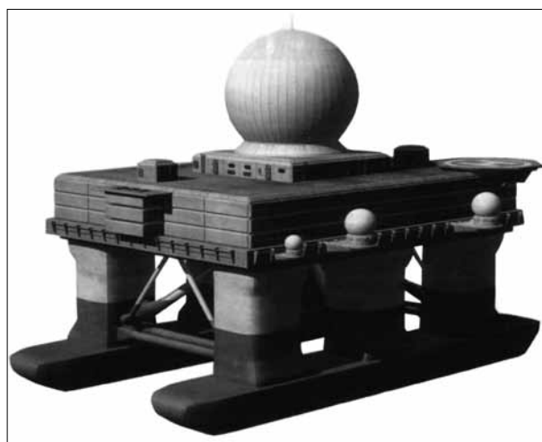
Рис. 2. Перспективная морская подвижная платформа континентальной ПРО
