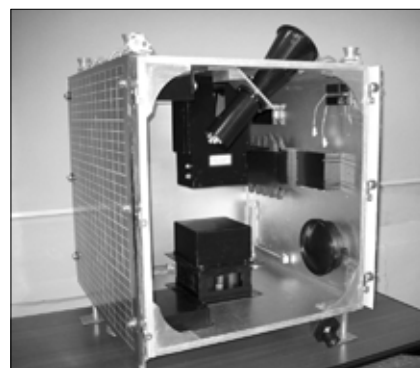
Baumanets (Ун-тет Баумана)
